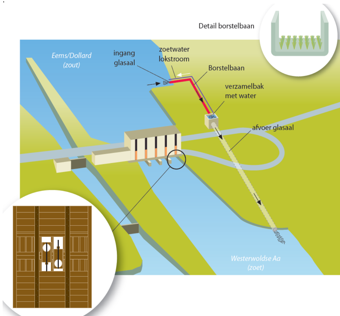
Vispassage Nieuwe Statenzijl
